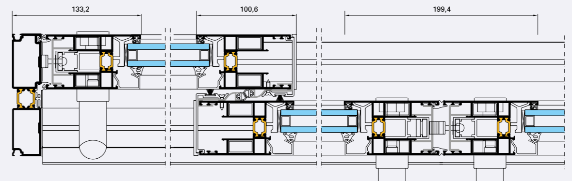
4 VANTAUX - 2 RAILS
