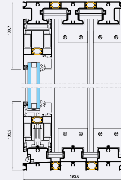
3 VANTAUX - 3 RAILS
