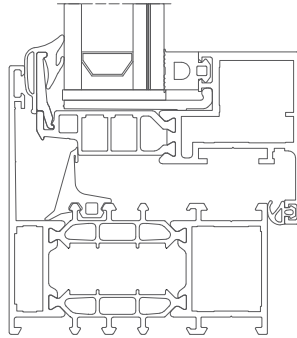
Avantis 75 HV Basic - Afgebeelde profiel combinatie: U_f = 2,05 \text{ W/m}^2\text{K}
