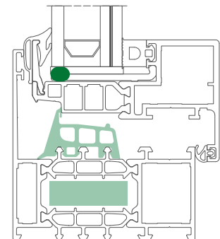
Avantis 75 SHI - Afgebeelde profiel combinatie: U_f = 1,71 \text{ W/m}^2\text{K}
