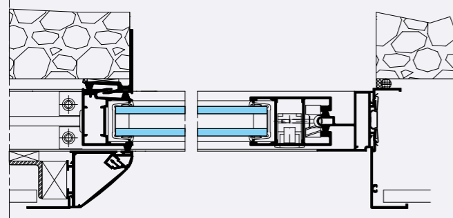
GALANDAGE MONORAIL - 1 VANTAIL
