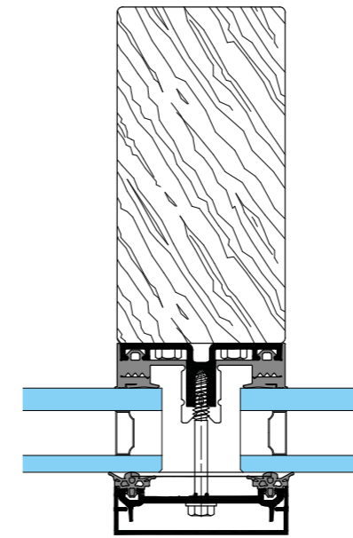
Structure bois La jonction des 2 matériaux doit répondre à des exigences spécifiques - nous consulter
