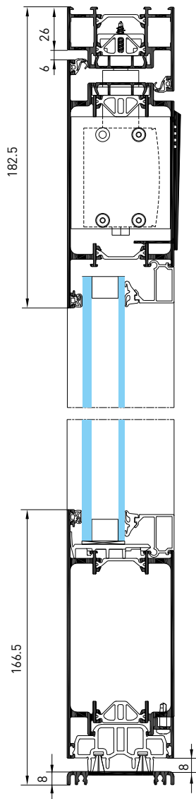
Coupe verticale seuil plat
