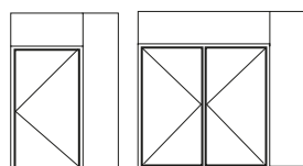
Ensemble menuisé, composé par empilage avec imposte et/ou fixes latéraux
