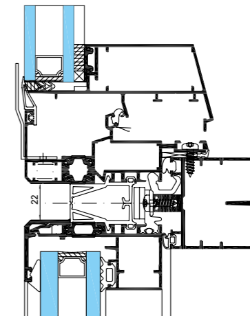
GEODE VEP ventana oculta oscilobatiente
