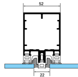
GEODE vidrio simple trama horizontal
