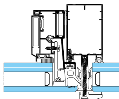
Ventana oculta italiana, trama horizontal
