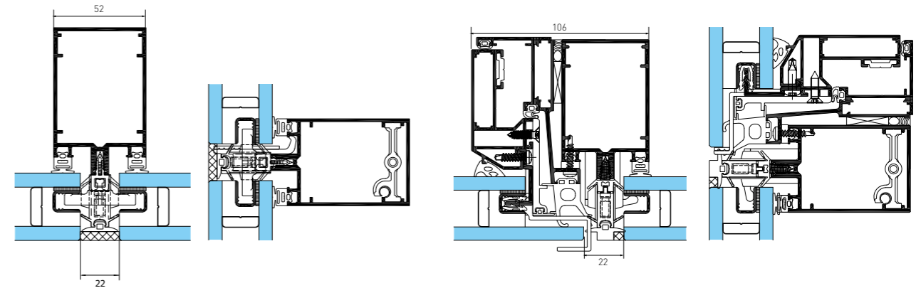
Ventana italiana o paralela
