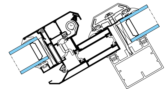
GEODE Ventana techo
