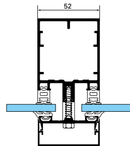
GEODE vidrio simple parrilla tradicional
