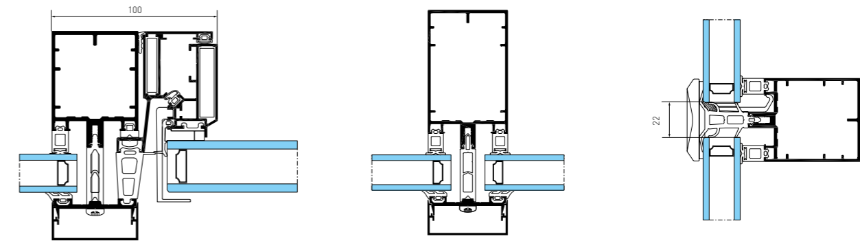
GEODE trama vertical con ventana oculta italiana
