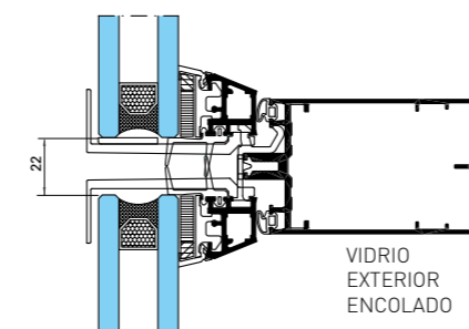
VIDRIO ESTRUCTURAL
