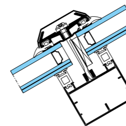
GEODE Techo, aspecto parrilla tradicional
