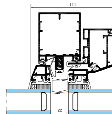
GEODE VEE ventana oculta italiana
