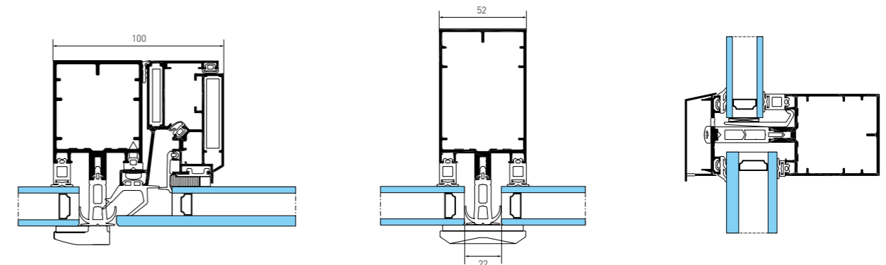
GEODE trama horizontal con ventana oculta italiana
