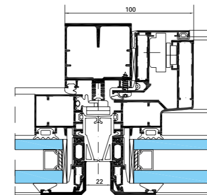
GEODE VEP ventana oculta italiana
