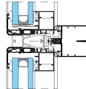
GEODE VEP ventana oculta italiana
