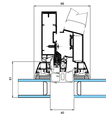
GEODE VEE ventana oculta oscilobatiente
