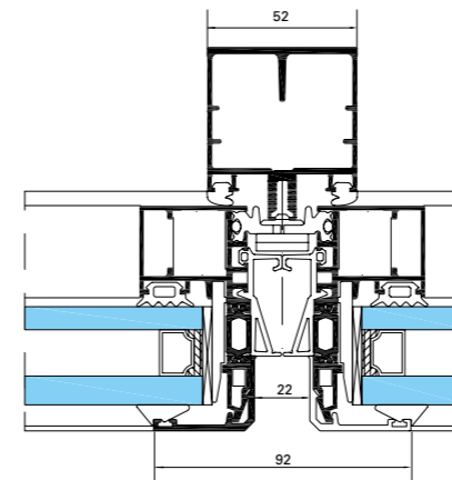
GEODE VEP visión partes fijas
