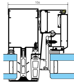
Ventana italiana
