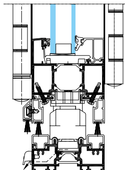
Ulos- ja sisäänavautuva: tuplaharjatiivisteellä.
