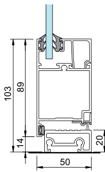
3 - Ovi huulostiivisteellä kynnystä vasten
