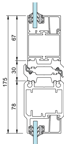
8 - Yläreuna, ovi yläosalla
