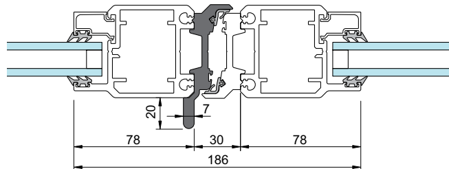
6 - Sisäänavautuvat pariovet, vahvistettu huullos käyntiovessa
