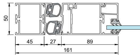
1 - Ovi sormisuojatulla takareunalla, kumilistat
