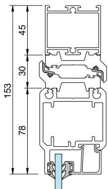
4 - Yläreuna, ovi karmilla
