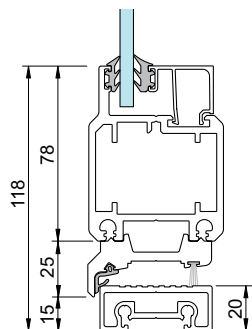
3 - Ovi huullostiivisteellä kynnystä vasten
