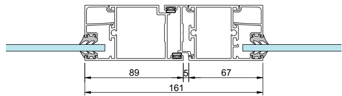
7 - Ovi vakioprofiililla ja sivuosalla
