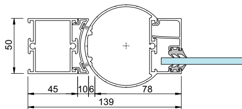
1 - Ovi sormisuojatulla takareunalla, pyöristetty alumiiniprofiili
