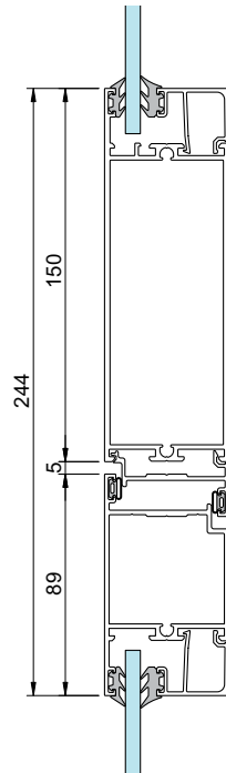
8 - Yläreuna, ovi yläosalla ja profiililla suurelle kääntöoviautomaatikalle
