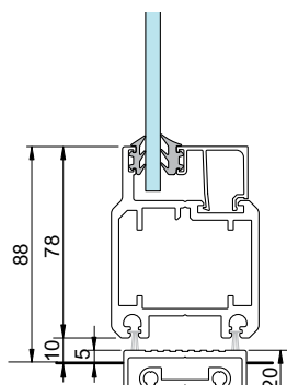
3 - Ovi upotetulla kynnyksellä
